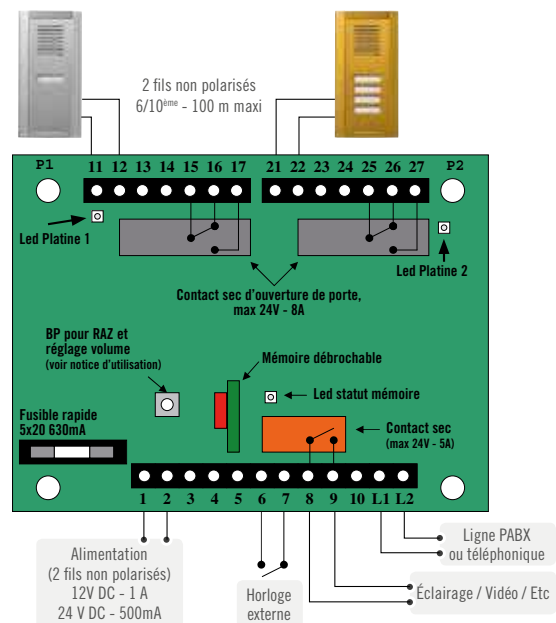
BRANCHEMENT 12/24V
