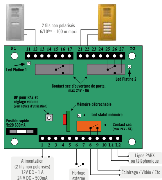
BRANCHEMENT 12/24V
