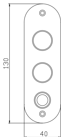
➤ Face avant
